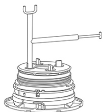
lösen der Abstandshalter
